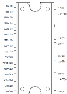
PIN1-PIN25
