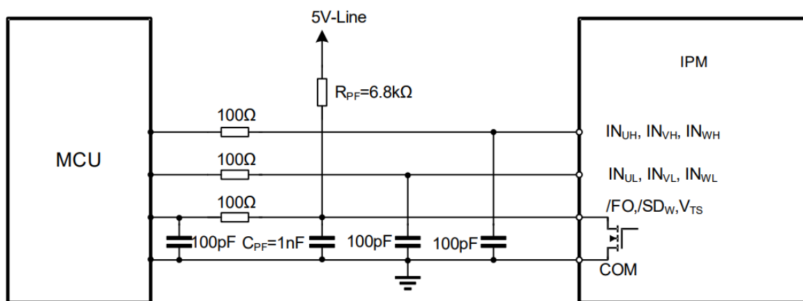
图 11. 推荐的 MCU I/O 接口电路
