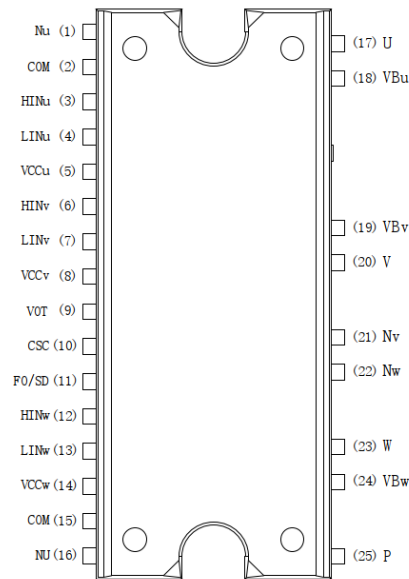
图 2：模块引脚分布示意图
